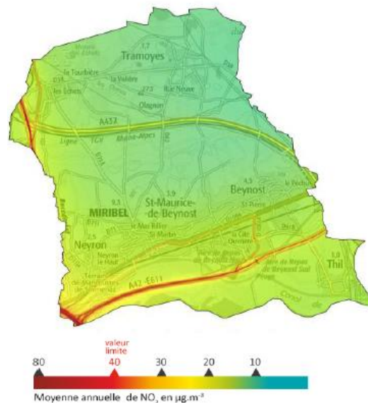
Figure 9: Carte d'exposition au dioxyde d'azote en 2016 sur le territoire.
