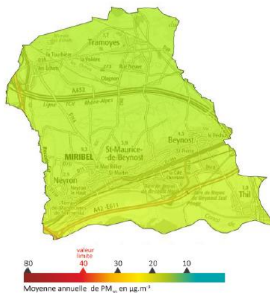
Figure 7 : Carte d'exposition aux PM10 sur le territoire en 2016.
