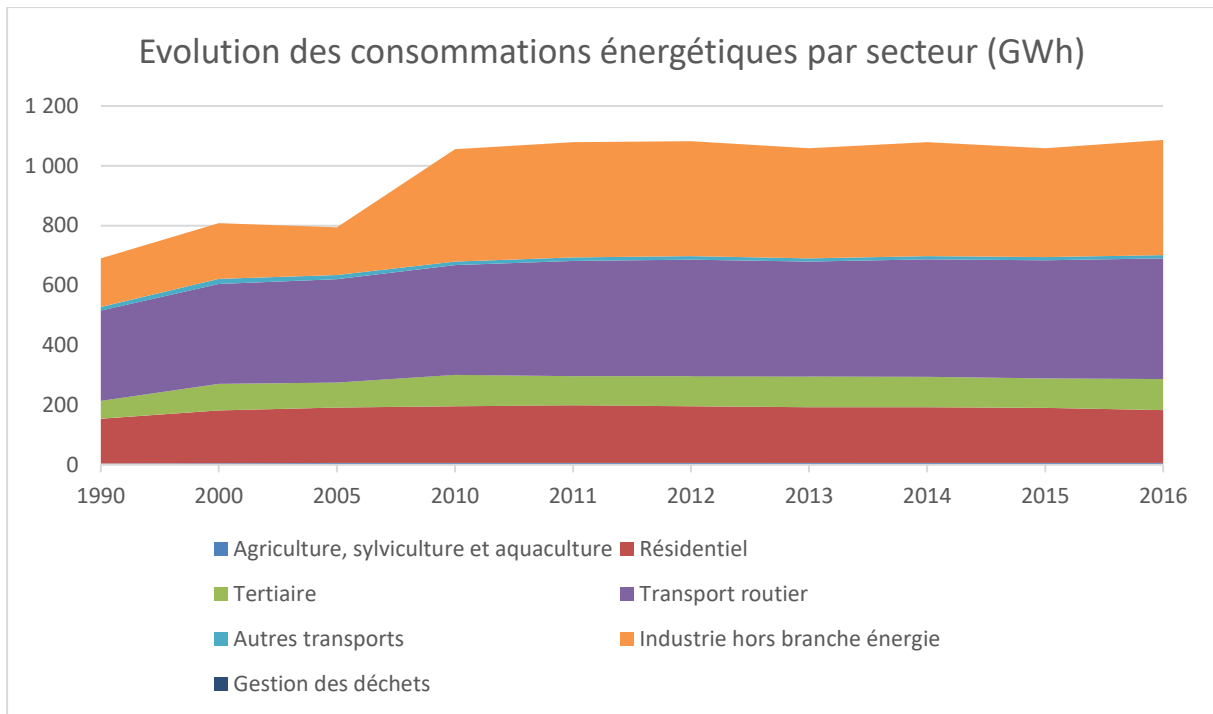
Figure 2 : Evolution des consommations énergétiques.
