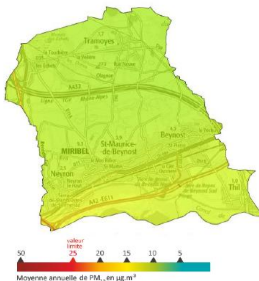
Figure 8 : Carte d'exposition aux PM 2,5 en 2016 sur le territoire.
