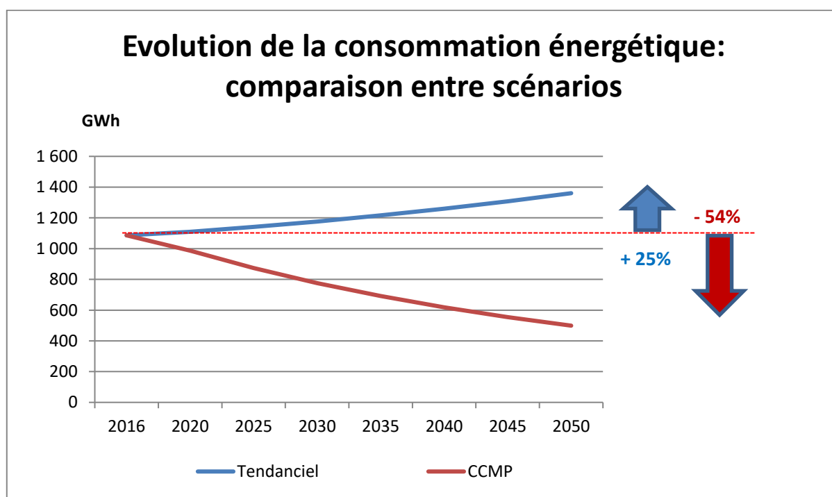
Evolution de la consommation énergétique : comparaison entre scénarios
